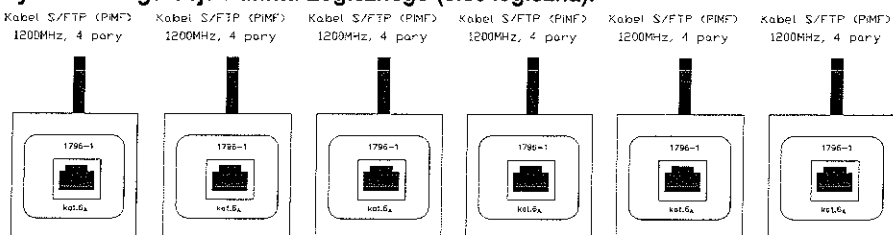
Rys. 6. Konfiguracja Punktu Logicznego (sieć logiczna).
